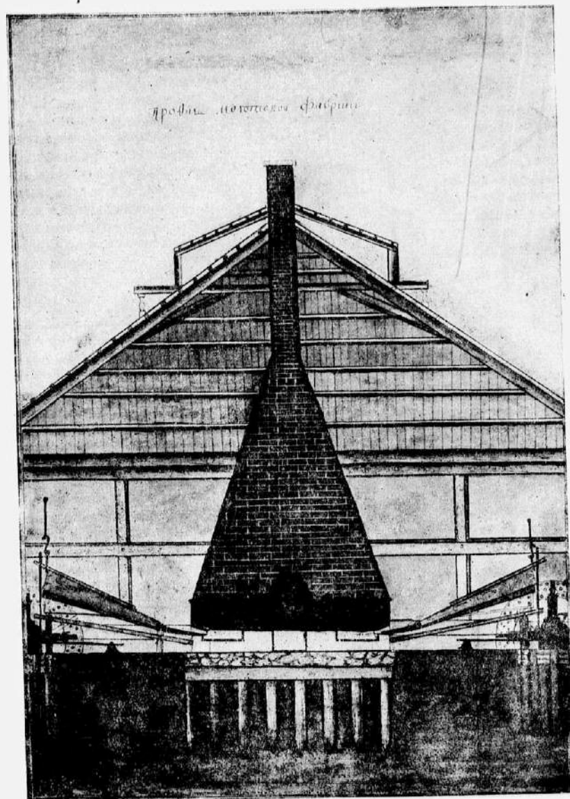
Профиль молотовой фабрики
